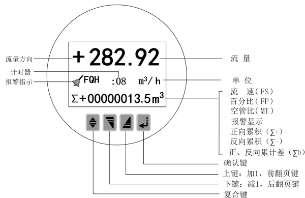
图 4.1.1 b 圆表键盘定义与液晶显示
