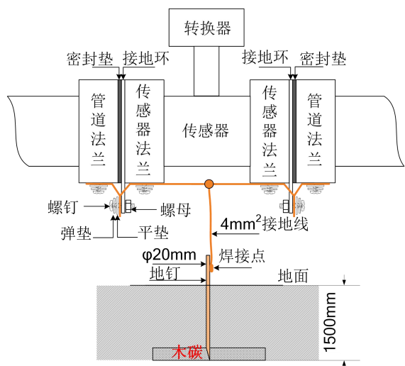
图 1.3.3 转换器接地示意图
