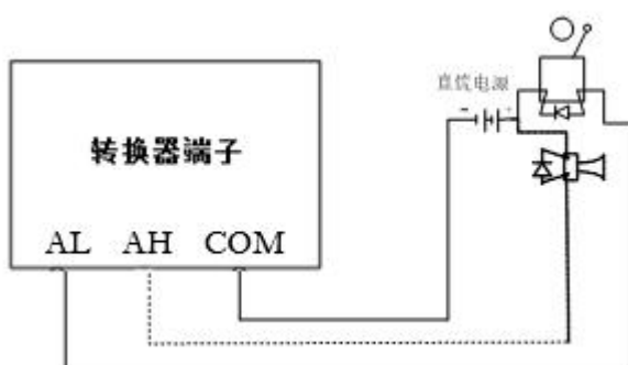
图 1.4.3 报警输出接线
