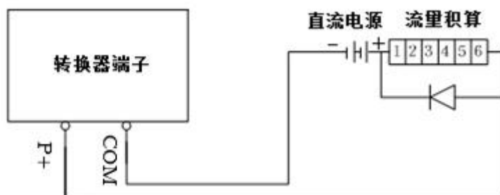
图 1.4.2 脉冲外供电源接电子计数器
