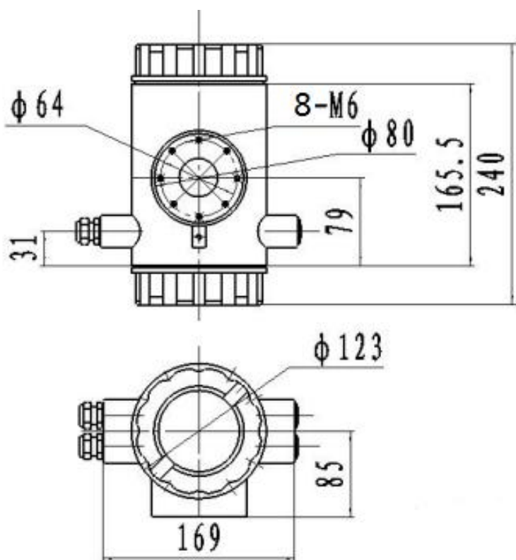
图 6.1 d 411B 壳外型尺寸图
