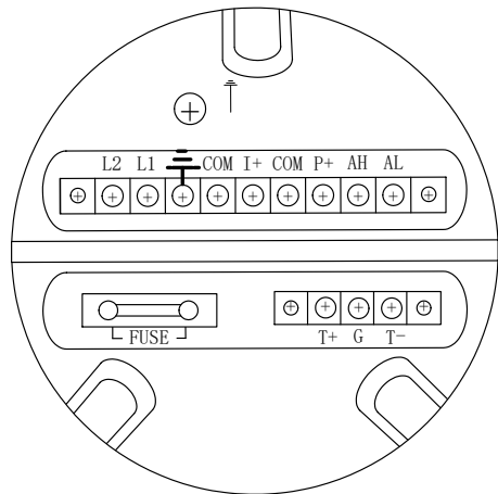
图 4.3.1c 圆表接线端子图
