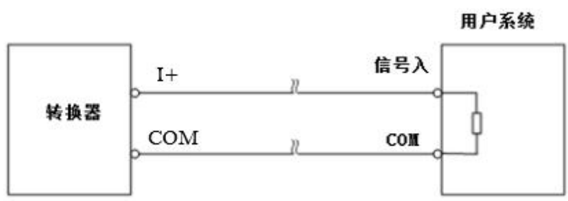
图 1.4.1 4~20mA 内供电接法（以 511B 壳体端子为例）
