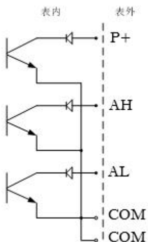
图 1.4.4 表内 OC 门连接方式（以 511B 壳体端子为例）
